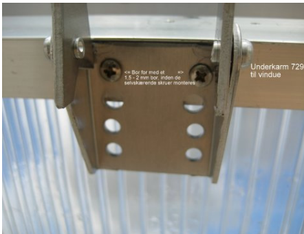
1: Bor for med et 2,0 mm bor
